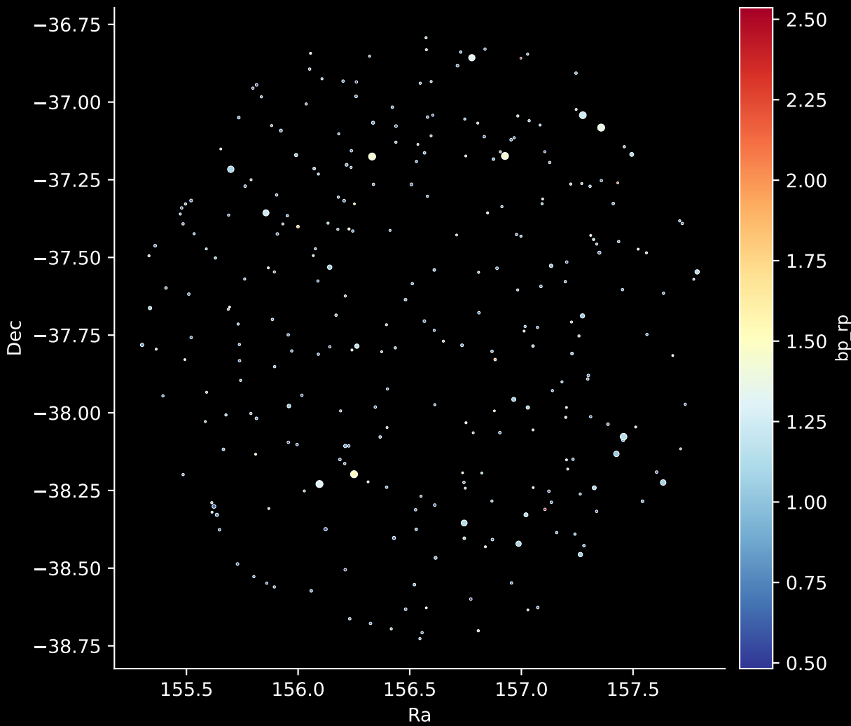
GALAH DR4 Field: [6951] Stars: 289
