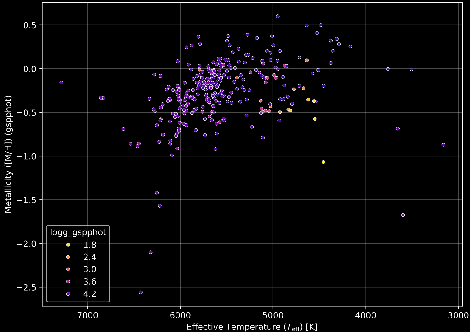
GALAH DR4 Field: [6951] Stellar Population Parameters (n= 289)
